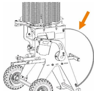
Ramię w pozycji niebezpiecznej (naciągniętej)
