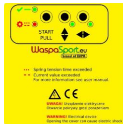
Panel sterownika WSPACON 3F dla wyrzutni 400V
